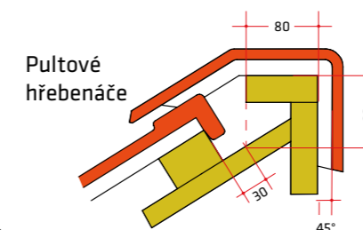
Řez střešním pláštěm.
